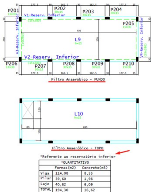
PLANTA DE FORMAS DA EST RESERVATÓRIO INFERIOR ESC 1:50
